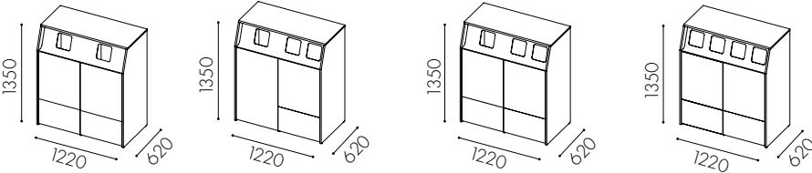
W3514 Dörr ovan till för 90 l kärl och lådutdrag undertill ** W3515 Hel dörr till vänster för rullkärl 140 l *, dörr ovan till för 2x60 kärl och lådutdrag undertill till höger ** W3516 Dörr ovan till för 90 l kärl i enkelt inkast, 2x60 i dubbelt inkast och lådutdrag undertill ** W3517 Dörr ovan till för 2x60 l kärl och lådutdrag undertill **
