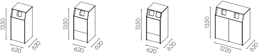
W3510 Hel dörr för rullkärl 140 liter * W3511 Dörr ovan till för 90 l kärl och lådutdrag undertill ** W3512 Dörr ovan till för 2x60 kärl och lådutdrag undertill ** W3513 Hela dörrar för rullkärl 140 liter *
