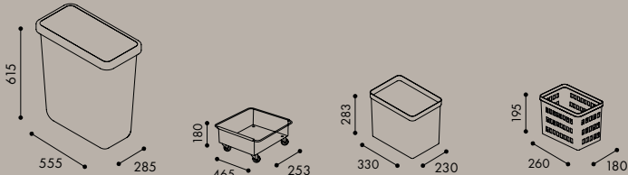
W0115 Kärl 60 liter Ett kärl ryms i varje utdragslåda W0116 Vagn 60 liter W0084 Kärl 19 liter W0145 Kompostkärl 8 liter
