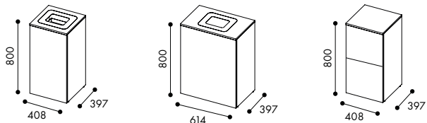
W3311 Hel dörr med säckhållare för 125 liters säck W3312 Hel dörr plats för 60 liters kärl W3313 2 lådor med plats för ett 19 l kärl per låda
