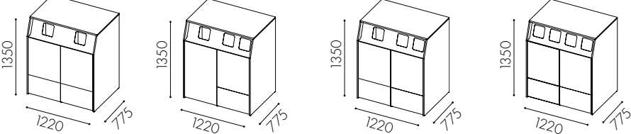
W3522 Dörr ovan till för 90 l kärl och lådutdrag undertill ** W3523 Hel dörr till vänster för rullkärl 1 l *, dörr ovan till för 2x60 kärl och lådutdrag undertill till höger ** W3524 Dörr ovan till för 90 l kärl i enkelt inkast, 2x60 i dubbelt inkast och lådutdrag undertill ** W3525 Dörr ovan till för 2x60 l kärl och lådutdrag undertill **
