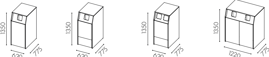
W3518 Hel dörr för rullkärl 190 liter * W3519 Dörr ovan till för 90 l kärl och lådutdrag undertill ** W3520 Dörr ovan till för 2x60 kärl och lådutdrag undertill ** W3521 Hela dörrar för rullkärl 190 liter *
