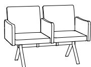
balk 2a 2 x 1-sits + klädda armstöd H 830 SH 450 B 1150 D 640
