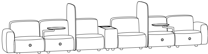
H 1200 SH 420 B 5385 D 880
