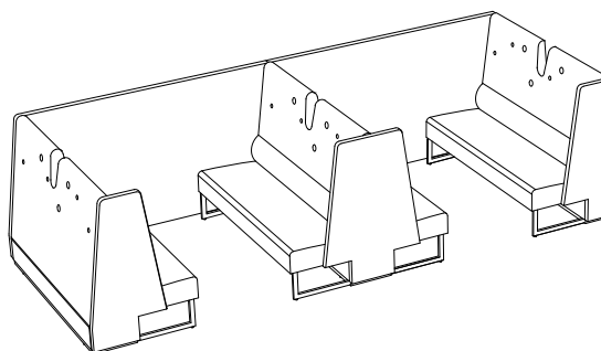
SA300 rak rygg väggställd (3) x 1 rak rygg (1) x 2 SA310 låg rak sits (4) x 4 SA350 kupévägg vänster (18) x 1 kupévägg rak (17) x 1 SA320 gavel enkel (10) x 1 gavel dubbel (11) x 1 gavel väggställd (12) x 1
