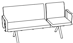
balk 3a 1 x 2-sits + 1 x 1-sits + metallarmstöd H 830 SH 450 B 1790 D 640
