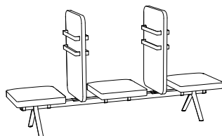
balk 3a + 2 3 x bänksits + 2 x skärmar med tidskriftsställ (dubbelsidigt) H 1260 SH 450 B 2340 D 520
