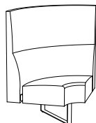
SA640 H 1230 SH 450 B 815 D 815
