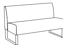
SA620 H 795 SH 450 B 1310 D 630
