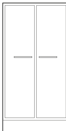
BD8/15 1580 x 800 x 372
