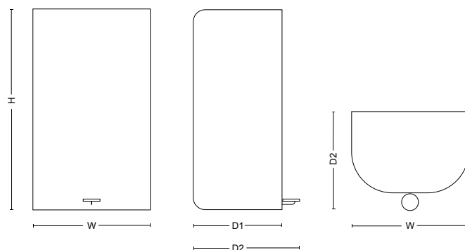
Pelican L H 800 mm, W 510 mm, D1 340 mm, D2 404 mm Art.nr. 262xx
