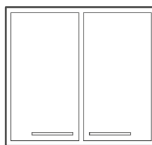
VD8/7 726 x 800 x 372
