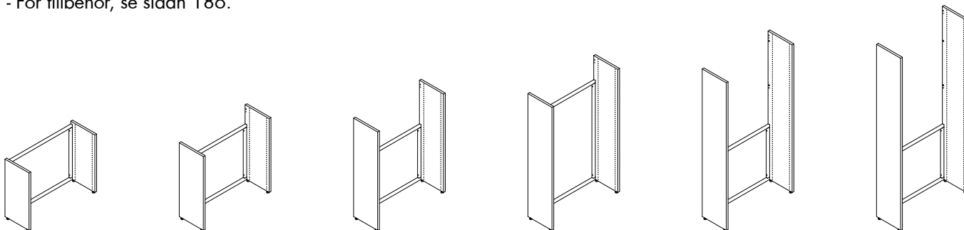
Enkelsidig fristående sektion - H720/920/1220/1520/1820/2120 mm
