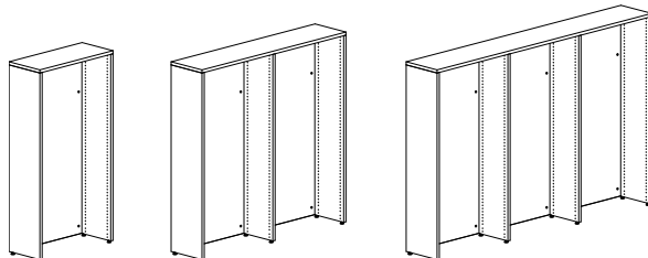
Enkel-/dubbelsidiga H1520 mm - 1/2/3 sektioner
