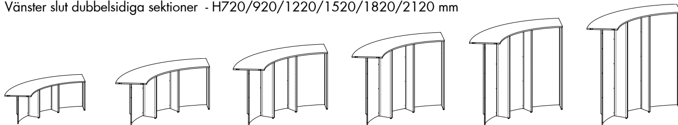
Höger slut dubbelsidiga sektioner - H720/920/1220/1520/1820/2120 mm
