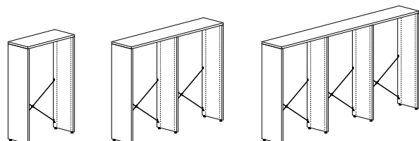
Enkel-/dubbelsidiga H 1220 mm - 1/2/3 sektioner
