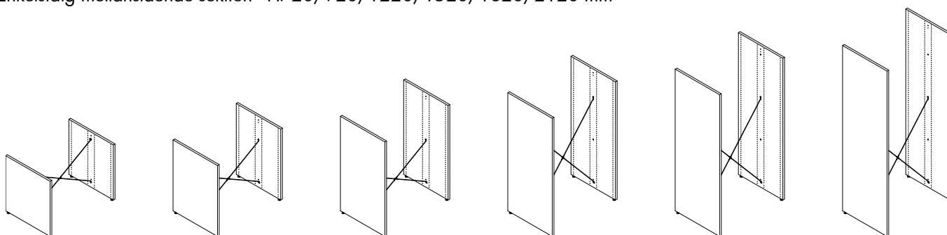
Dubbelsidig fristående sektion - H720/920/1220/1520/1820/2120 mm
