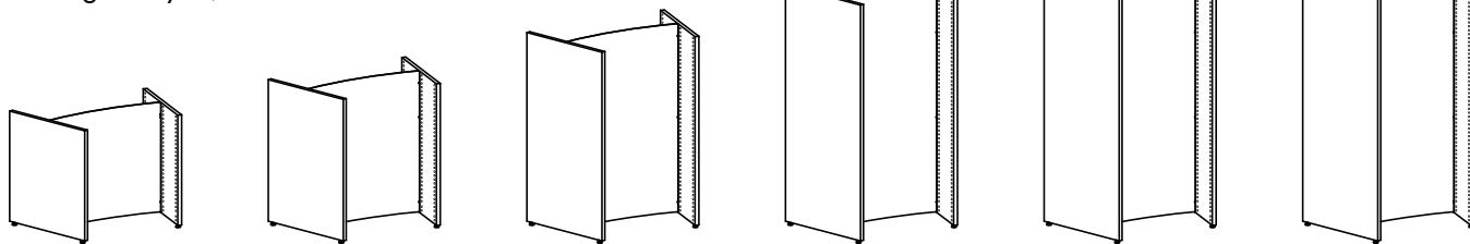
Dubbelsidig fristående sektion - H720/920/1220/1520/1820/2120 mm
