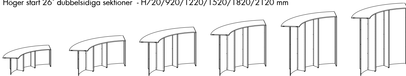
Mellan 26° dubbelsidiga sektioner - H720/920/1220/1520/1820/2120 mm
