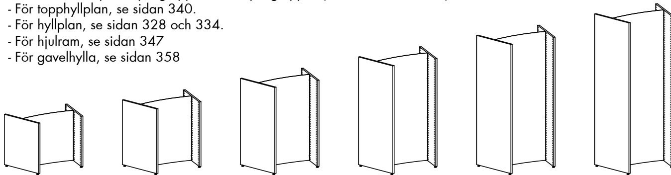
Dubbelsidig fristående sektion - H720/920/1220/1520/1820/2120 mm
