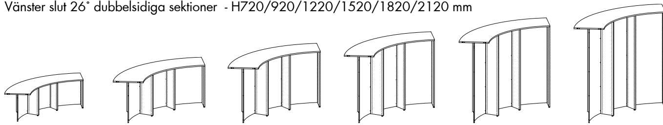
Höger slut 26° dubbelsidiga sektioner - H720/920/1220/1520/1820/2120 mm
