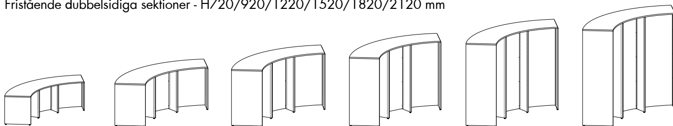
Vänster start dubbelsidiga sektioner - H720/920/1220/1520/1820/2120 mm
