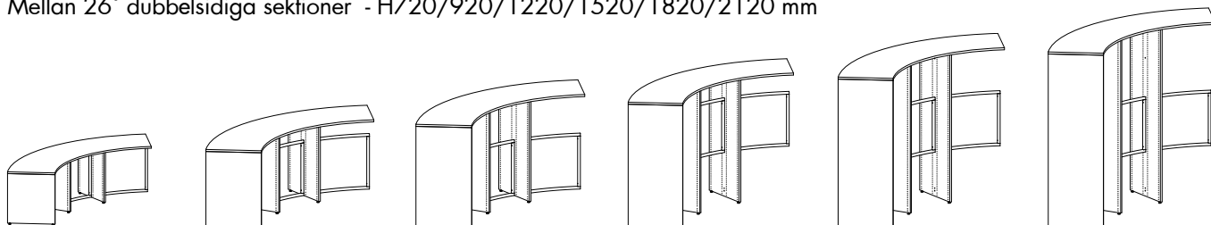
Vänster slut 26° dubbelsidiga sektioner - H720/920/1220/1520/1820/2120 mm
