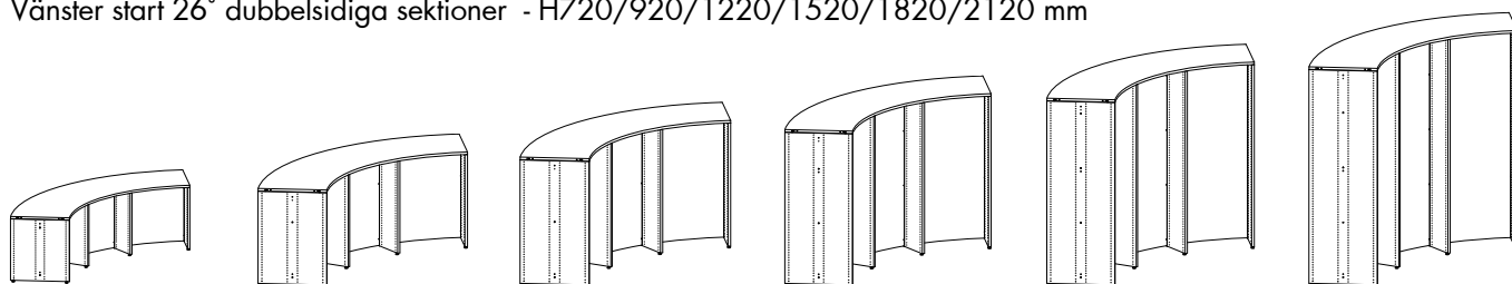
Höger start 26° dubbelsidiga sektioner - H720/920/1220/1520/1820/2120 mm
