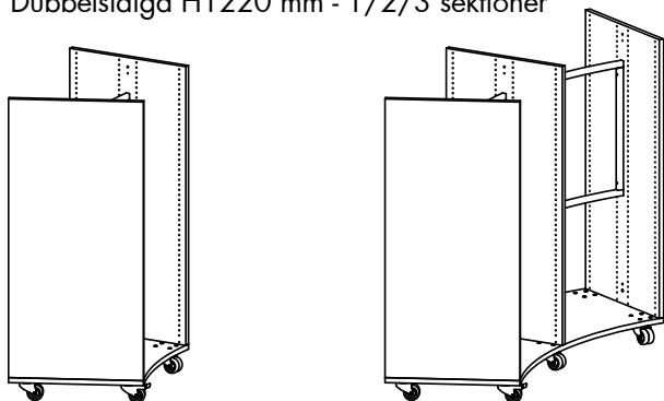
Dubbelsidiga H1520 mm - 1/2/3 sektioner
