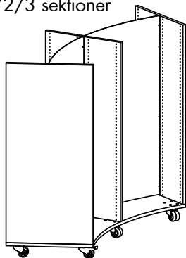
Dubbelsidiga H1520 mm - 1/2/3 sektioner
