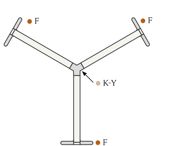
EXEMPEL (Koppling Y-120°)
