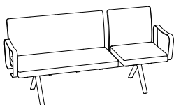
balk 3a 1 x 2-sits + 1 x 1-sits + metallarmstöd H 830 SH 460 B 1790 D 640
