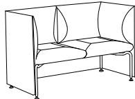
SA820 fristående (4) H 850 SH 450 B 1310 D 665
