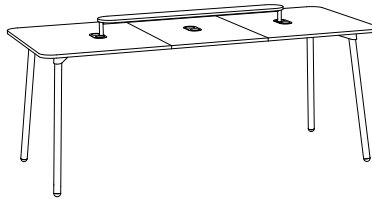
950x1200 x 2 + 750x1200 x 1 + hylla lång x 1 H skiva 1050 B 2650 D 1200
