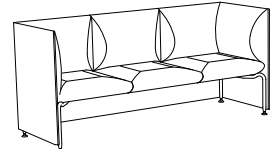
SA830 fristående (13) H 850 SH 450 B 1940 D 665
